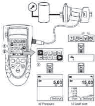
DPI880 外部智能压力模块压力及泄漏测试
