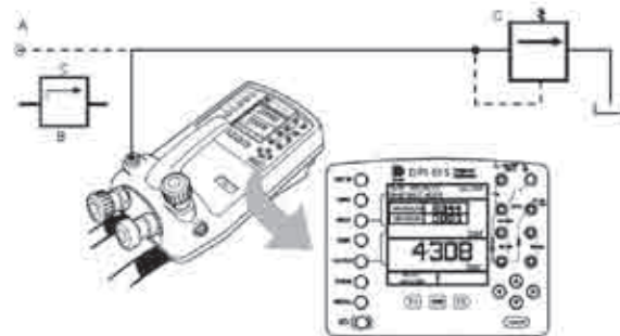
A- 外部压力源 (仅适用于指示仪型) C- 待测安全阀
