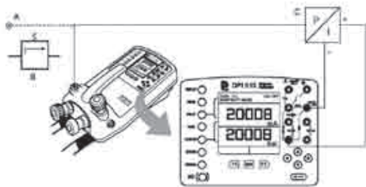
A- 外部压力源 (仅适用于指示仪型) C- 压力至电流 24V 设备
