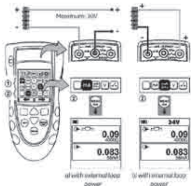
DPI880 功能区 2 测试 mA 信号，内部 / 外部供电
