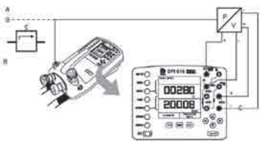
A- 外部压力源 (仅适用于指示仪型) C- 电源 10V
