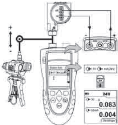
DPI800/802 校准两线制变送器，内部 24 伏供电
