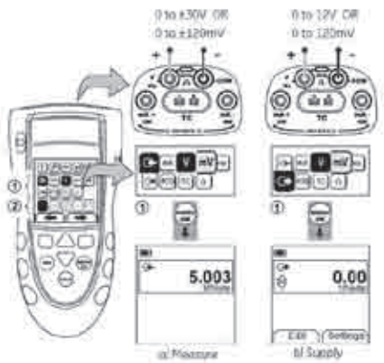
DPI880 功能区 1 测量及输出电压信号
