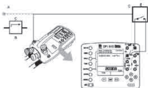
A- 外部压力源 (仅适用于指示仪型) B- 压力调节器 C- 待测压力开关
