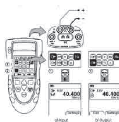
DPI880 测试与输出频率信号
